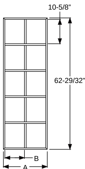
10-Lite (2264)
