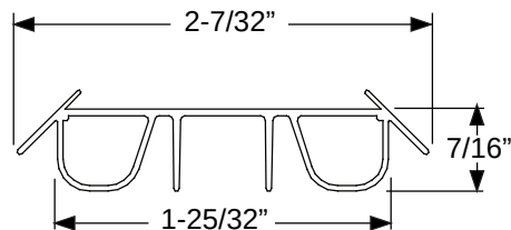
Dual Bulb No Kerf Door Bottom
