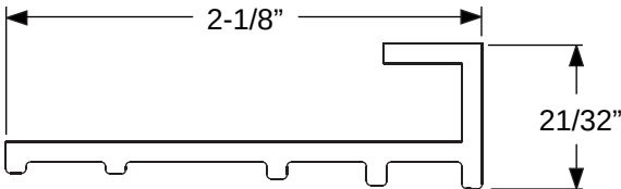
Sidelite Door Bottom - Aluminum Outswing Sill
