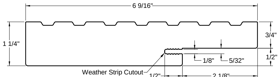
6-9/16" Jamb
