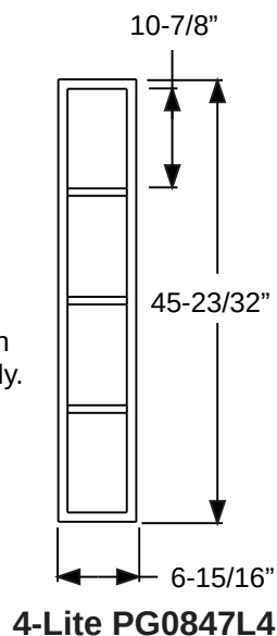
Muntin Bar
