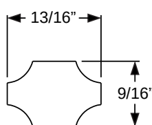
Muntin Bar
