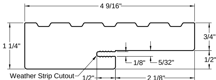
4-9/16" Jamb
