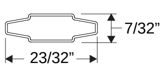
GBG Grille Section (Contour)
