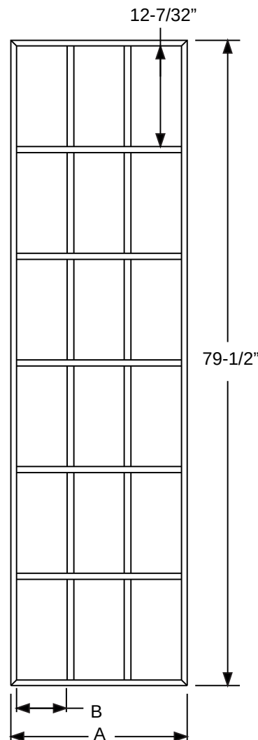
18 Lite
