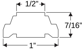
Muntin Bar
