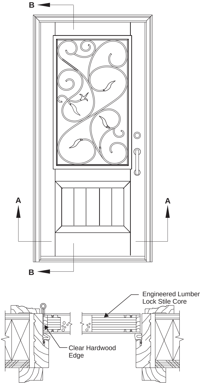
6/8 Single Door Inswing
