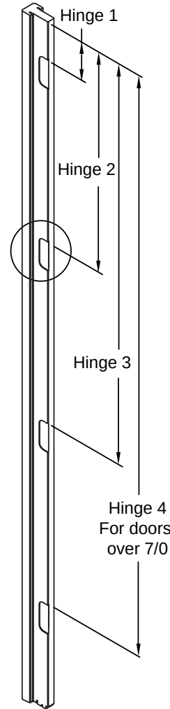
8/0 Jamb Shown
