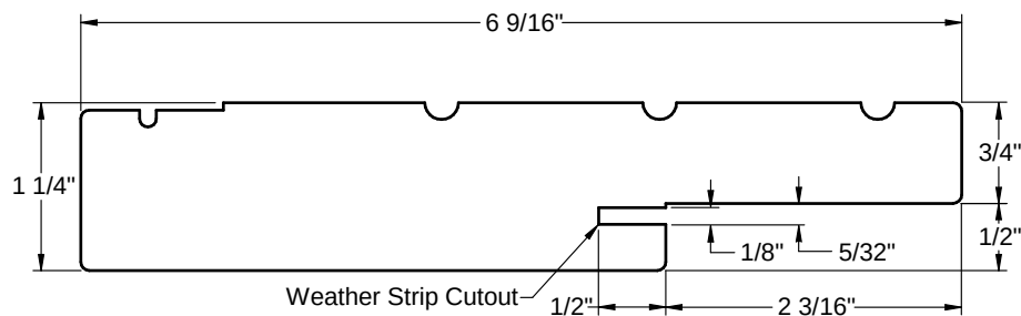
6-9/16" Jambs
