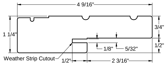
4-9/16" Jambs
